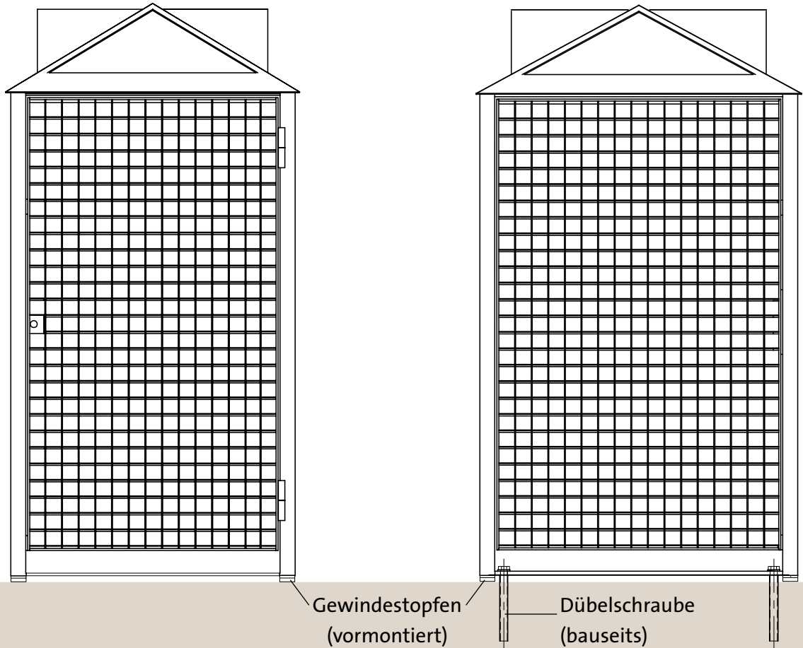
Vorderansicht Tür
