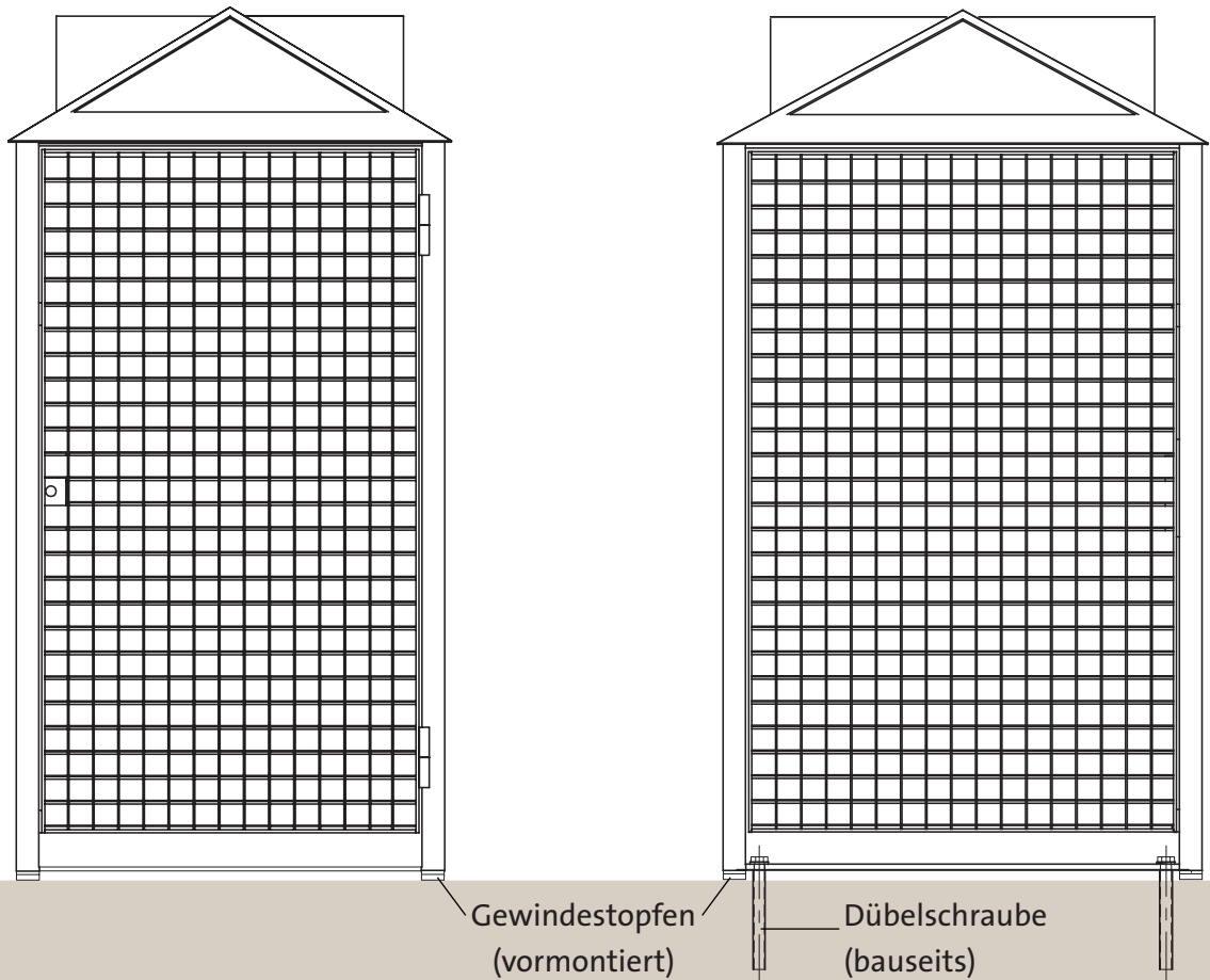
Vorderansicht Tür
